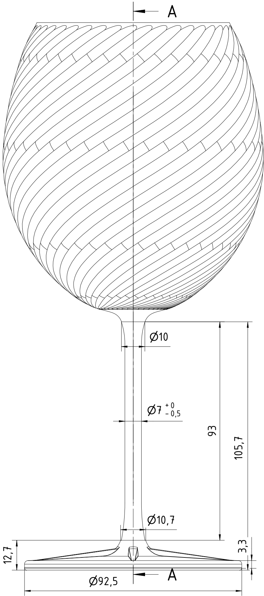
ANSICHT ( 1 : 2 )
